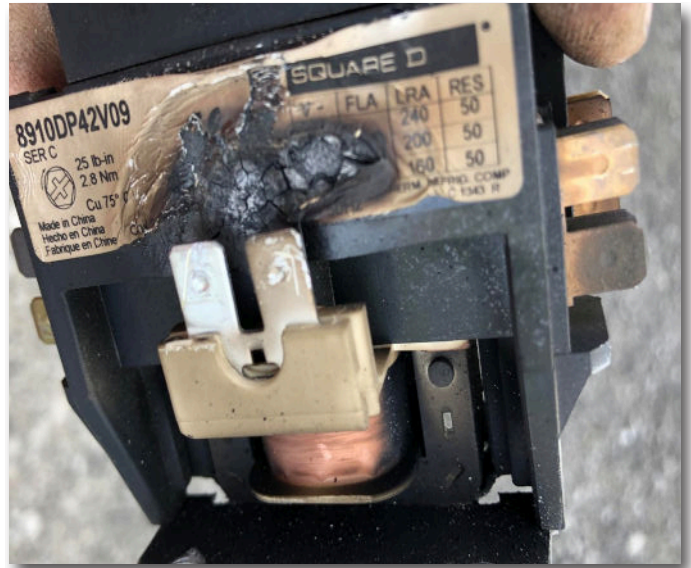
Sudden fault on a «TMR mixer» motor contactor.
